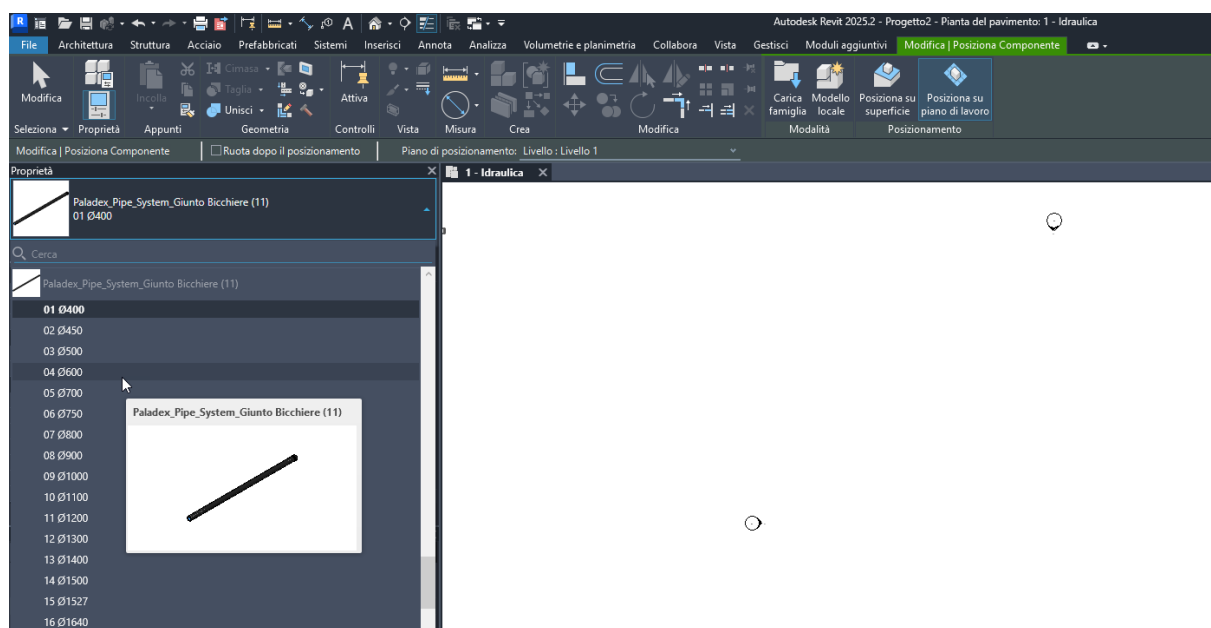
Figura 6– Inserimento e posizionamento della giunzione: selezione della tipologia e del diametro dal menu delle famiglie.
